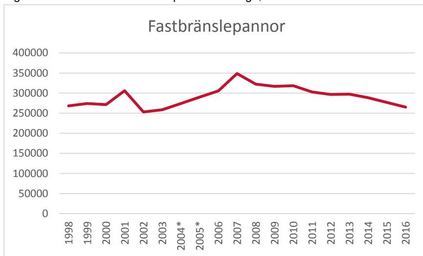
Figur 2 Beståndet av fastbränslepannor i Sverige, 1998–2016
