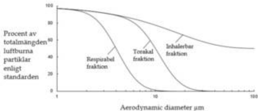
Figur 1. Inhalerbar, torakal och respirabel fraktion enligt konventionen i standarden SS-EN 481 angivna som procent av totalmängden luftburna partiklar.
